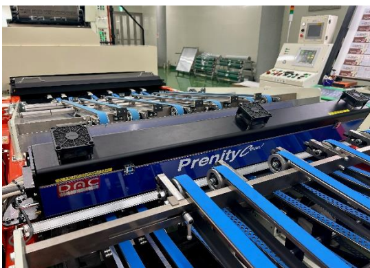
インラインカメラ（センサータイプ）
